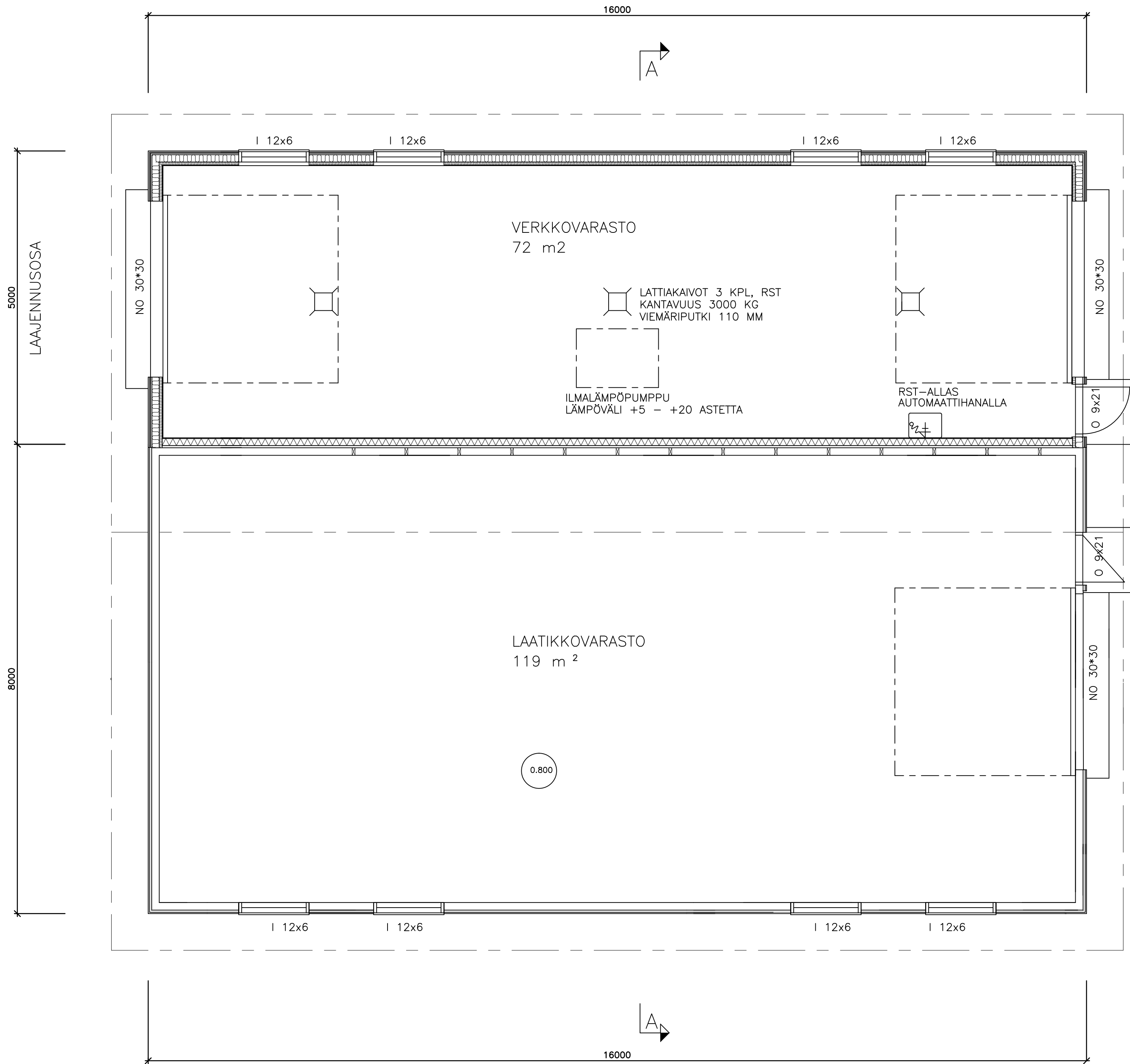
POHJAPIIRROS
